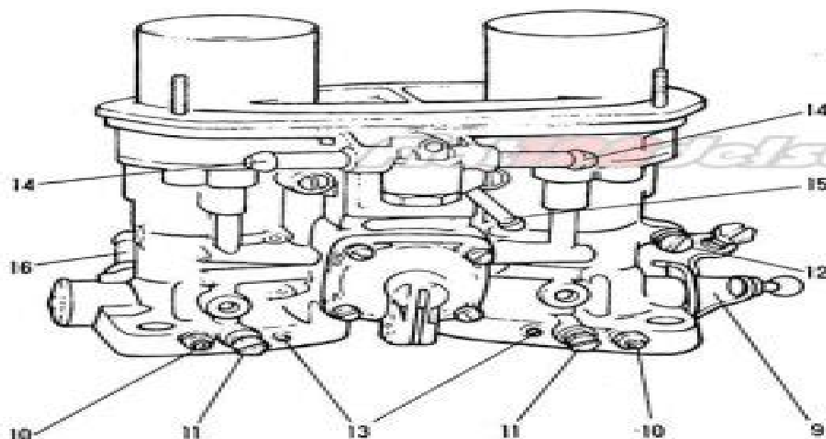
Fig. 2.- Carburador Weber 40 IDF 13.
