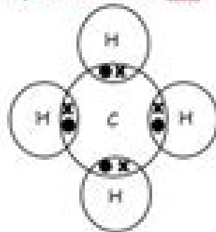
Methane ( \text{CH}_4 )
