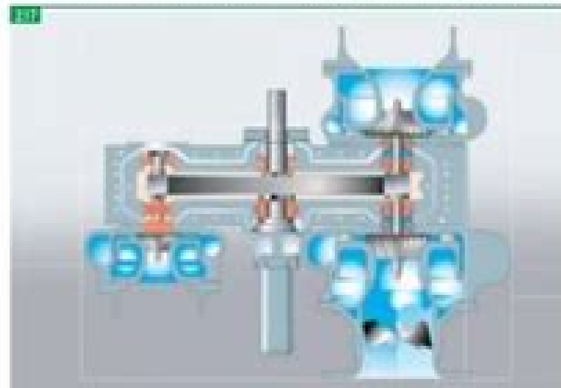
Compresor centrífugo de dos etapas con un eje de rotación.
