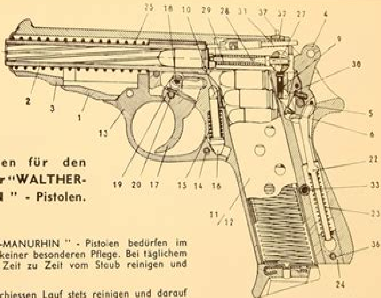
SCHNITT DURCH DIE "WALTHER-MANURHIN" - PISTOLE MOD. "PP"
