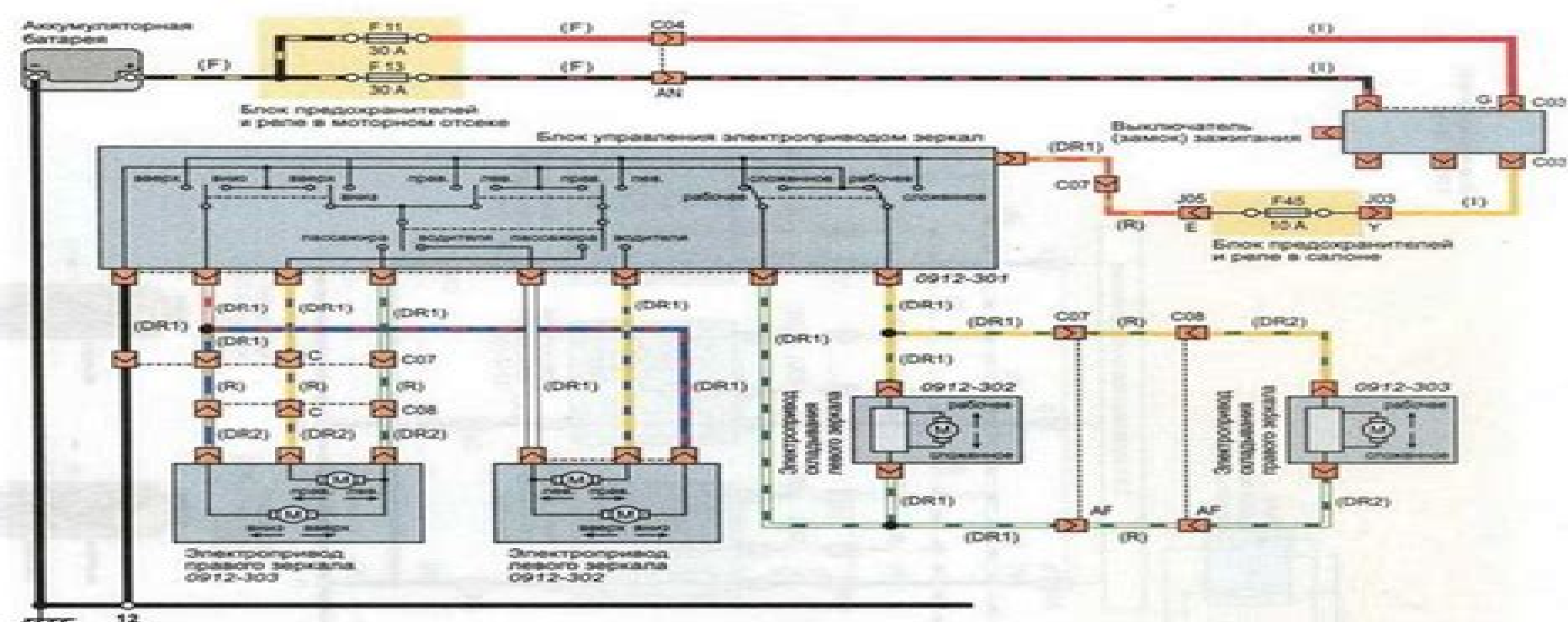
Блок управления электроприводом зеркал (DR1) 0912-301
