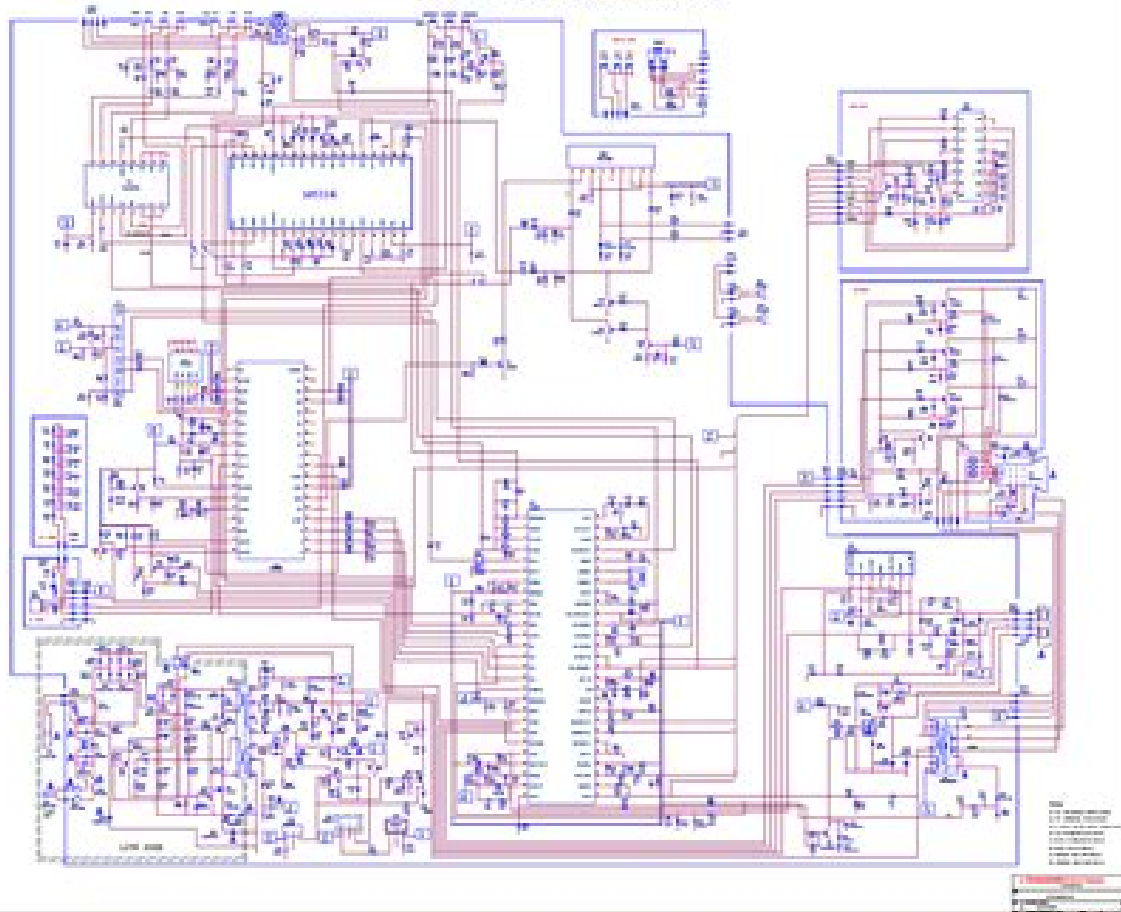
K05XAB1821 彩色电视机电路电源原理图
