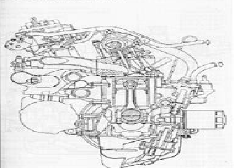
Fig. 26. Corte transversal del motor Tipo
