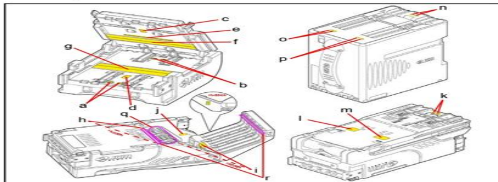
Figura 10 Ubicación de los sensores del iVIZION
