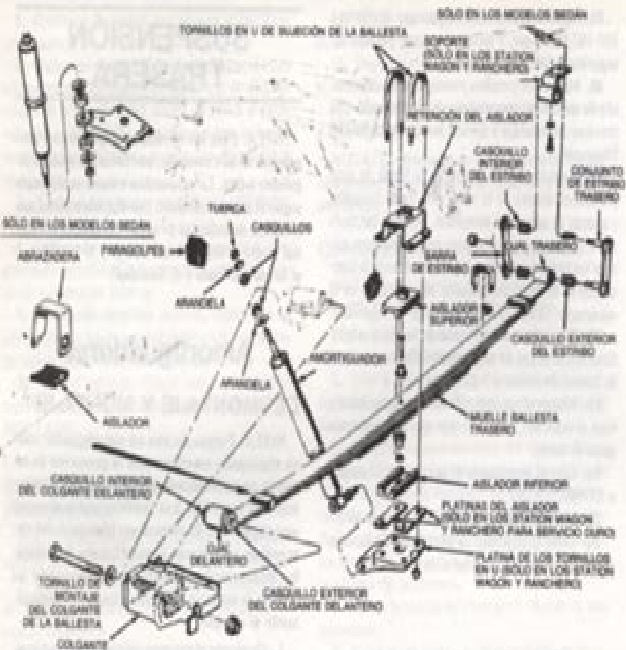
Vista en despiece ordenado de una suspensión trasera con muelle de ballesta de hojas
