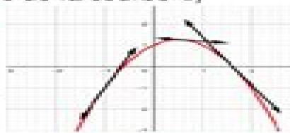
Graphique d'une fonction concave
