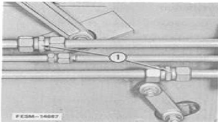
1. Tube nut
