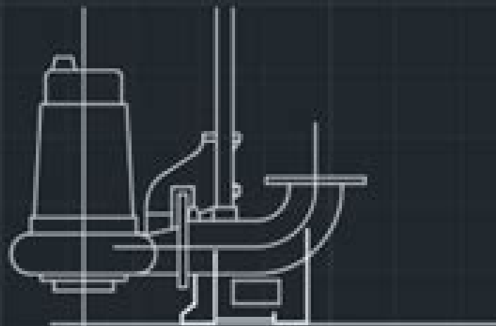
BOMBA FLYGT 3101 — ESC.~1:20
