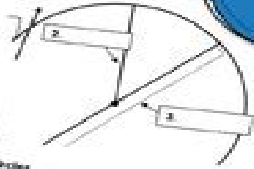
Secant Tangent
