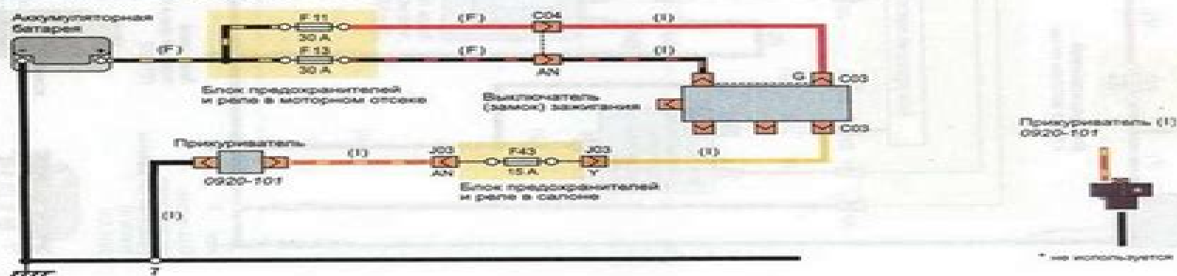
Схема 22. Прикуриватель
