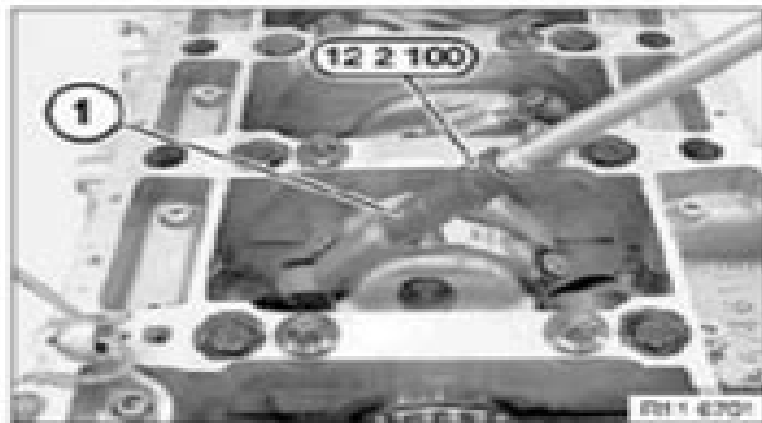
Fig. 156 : Retrait des boulons de bielle
