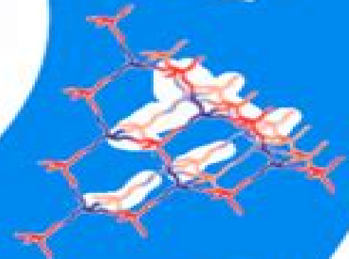
Tetra-PEG Gel
