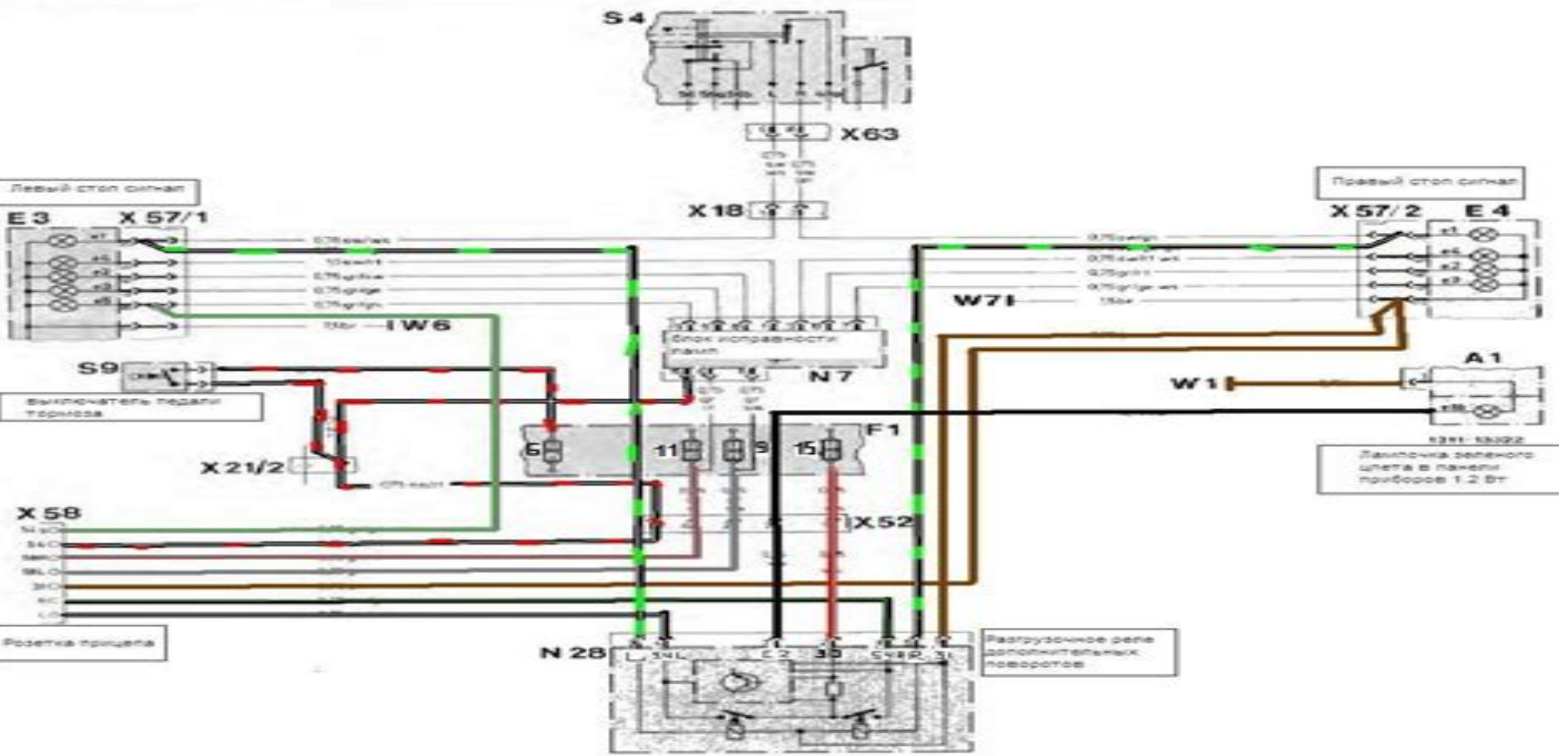
Schaltplan Anhängavorrichtung, Fahrzeuge ab ca. 9.85 bis ca. 7.86 mit Glühlampenausfallkontrolle ohne Dauerstromleitung Klemme 30
