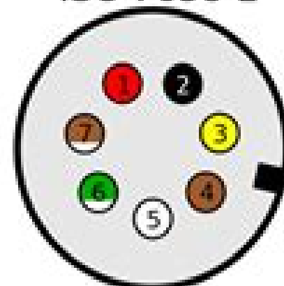
ISO 7638-2
