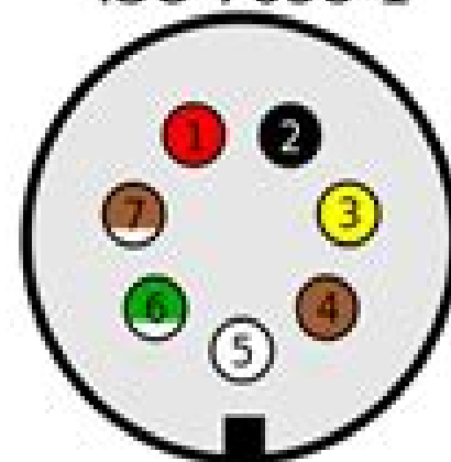
ISO 7638-1
