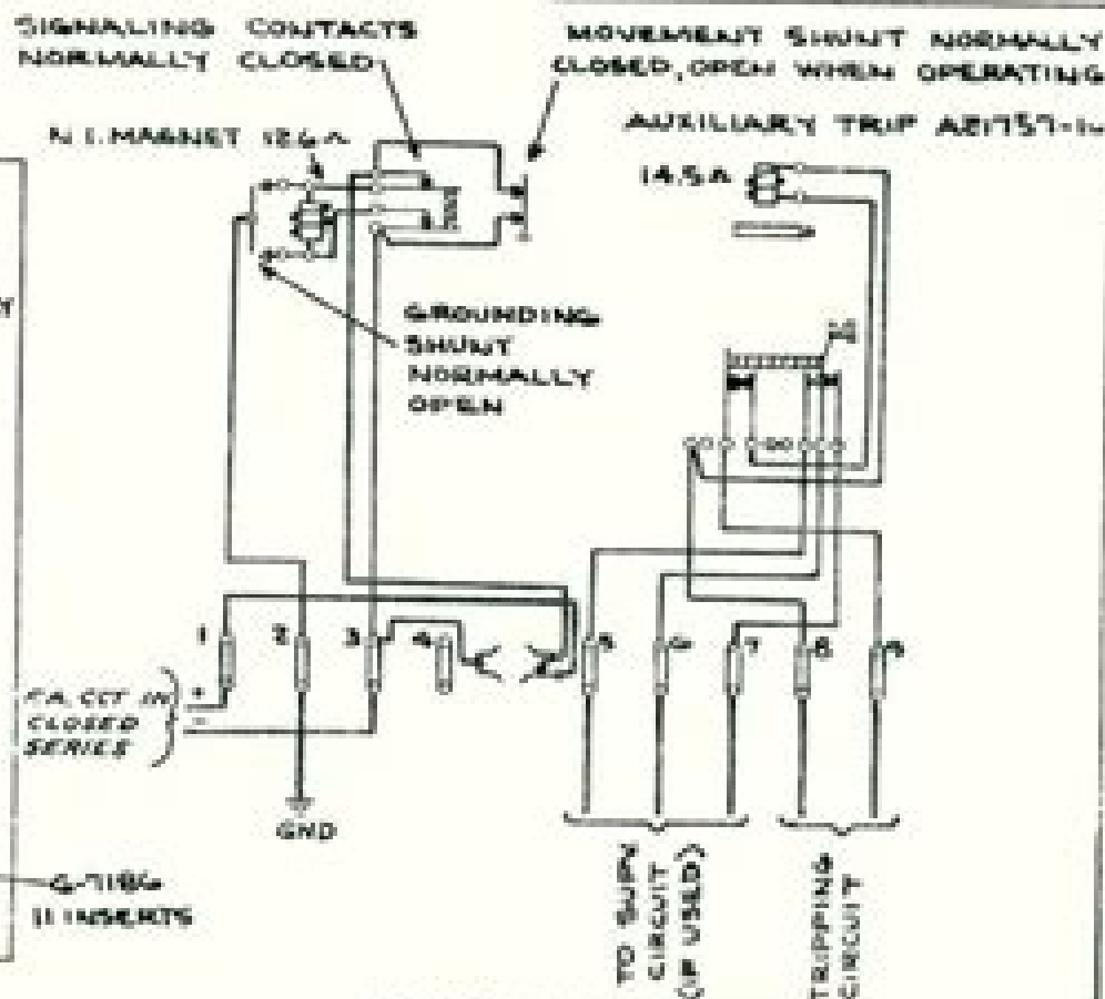
SCHEMATIC WIRING
