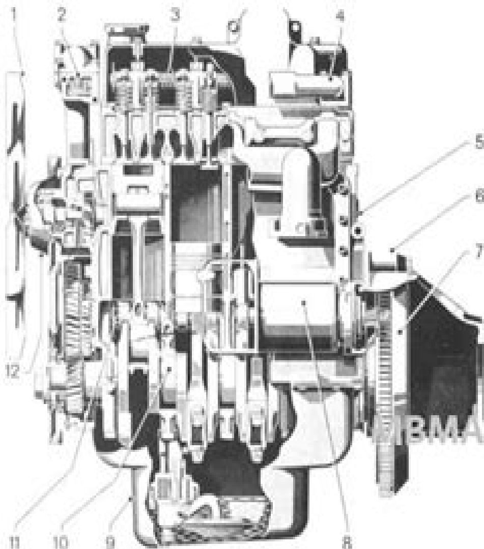
CORTE LONGITUDINAL
