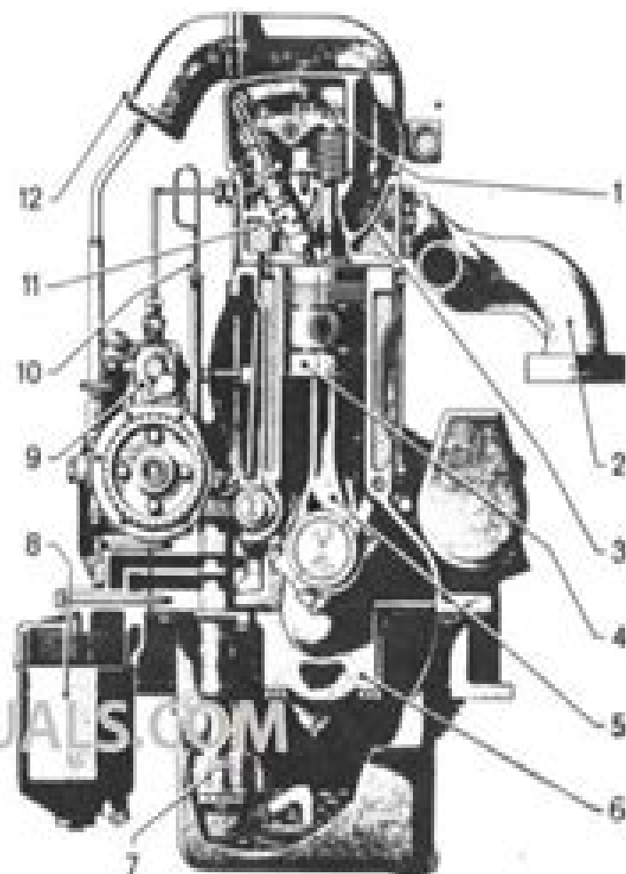
CORTE TRANSVERSAL
