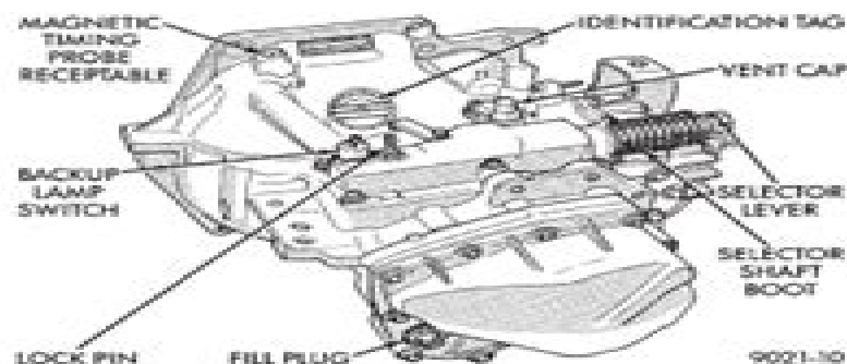
Fig. 1 Manual Transaxle Fill Plug
