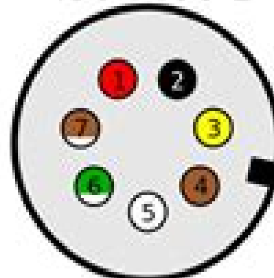
ISO 7638-2
