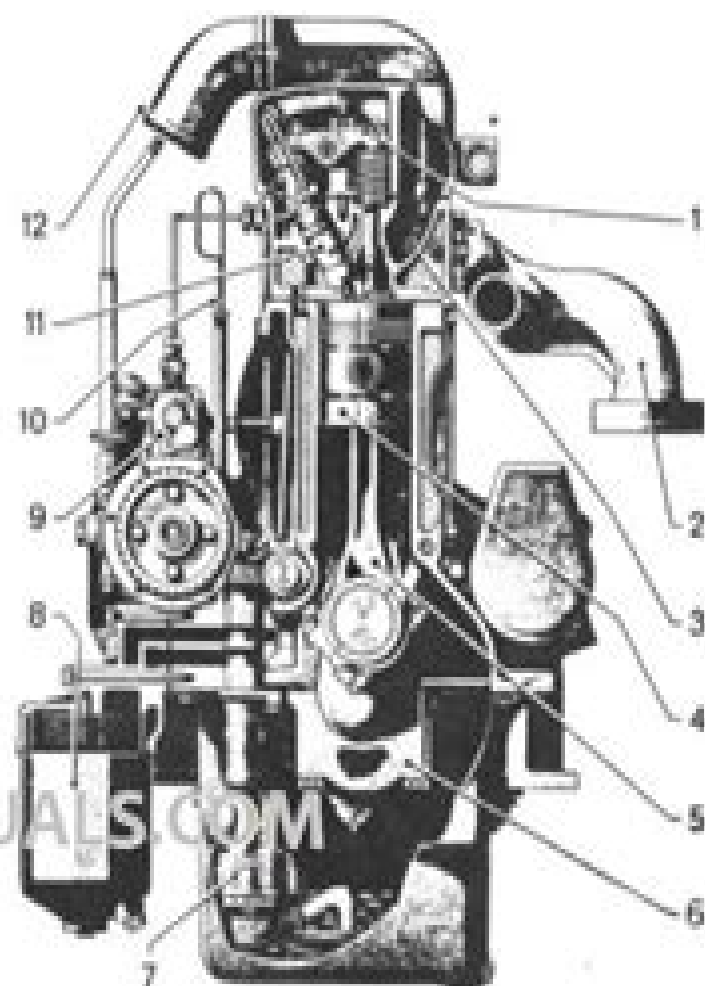
CORTE TRANSVERSAL
