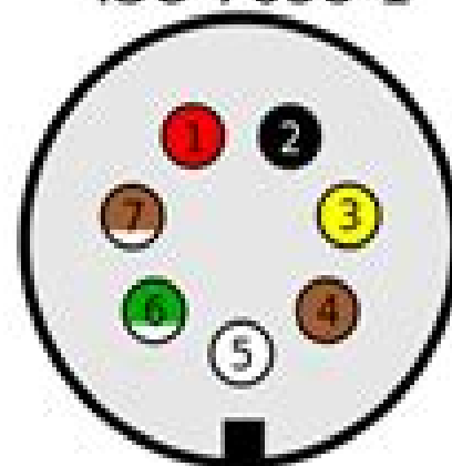
ISO 7638-1
