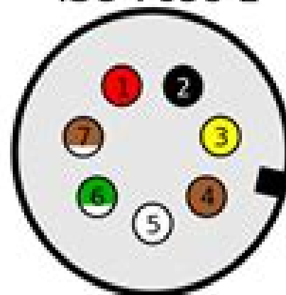
ISO 7638-2
