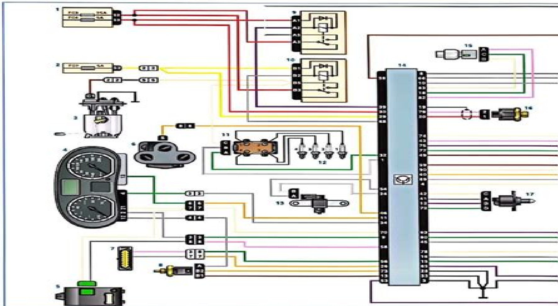
Diagrama del sistema de control electrónico del motor: 1 - caja de fusibles y relés en el compartimento del motor; 2 - caja de fusibles en el habitáculo; 3 - módulo de combustible; 4 - grupo de instrumentos; 5 - unidad de conmutación; 6 - unidad de control de ventilación, calefacción y aire acondicionado; 7 - conector de diagnóstico (bloque de diagnóstico); 8 - sensor de temperatura del refrigerante; 9 - relé principal; 10 - relé de potencia de la bomba de combustible y de la bobina de encendido; 11 - bobina de encendido; 12 - bujías; 13 - sensor de posición del cigüeñal; 14 - unidad de control del motor (ECU); 15 - sensor de temperatura del refrigerante; 16 - sensor de posición del cigüeñal; 17 - sensor de temperatura del refrigerante.
