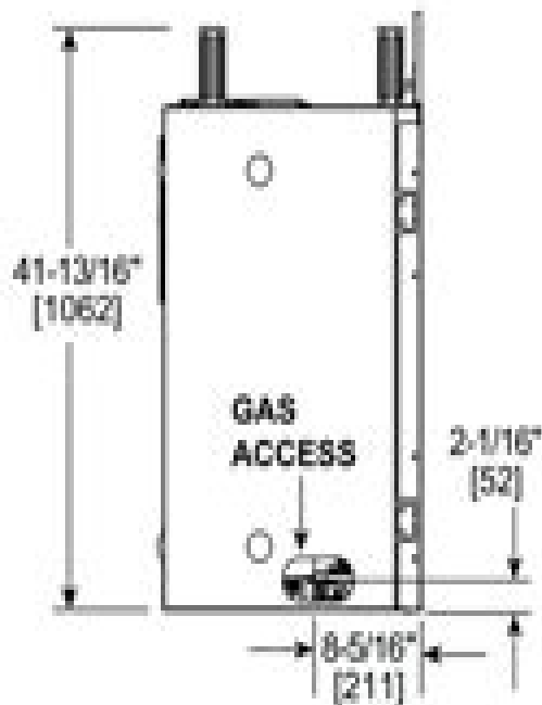
LEFT SIDE
