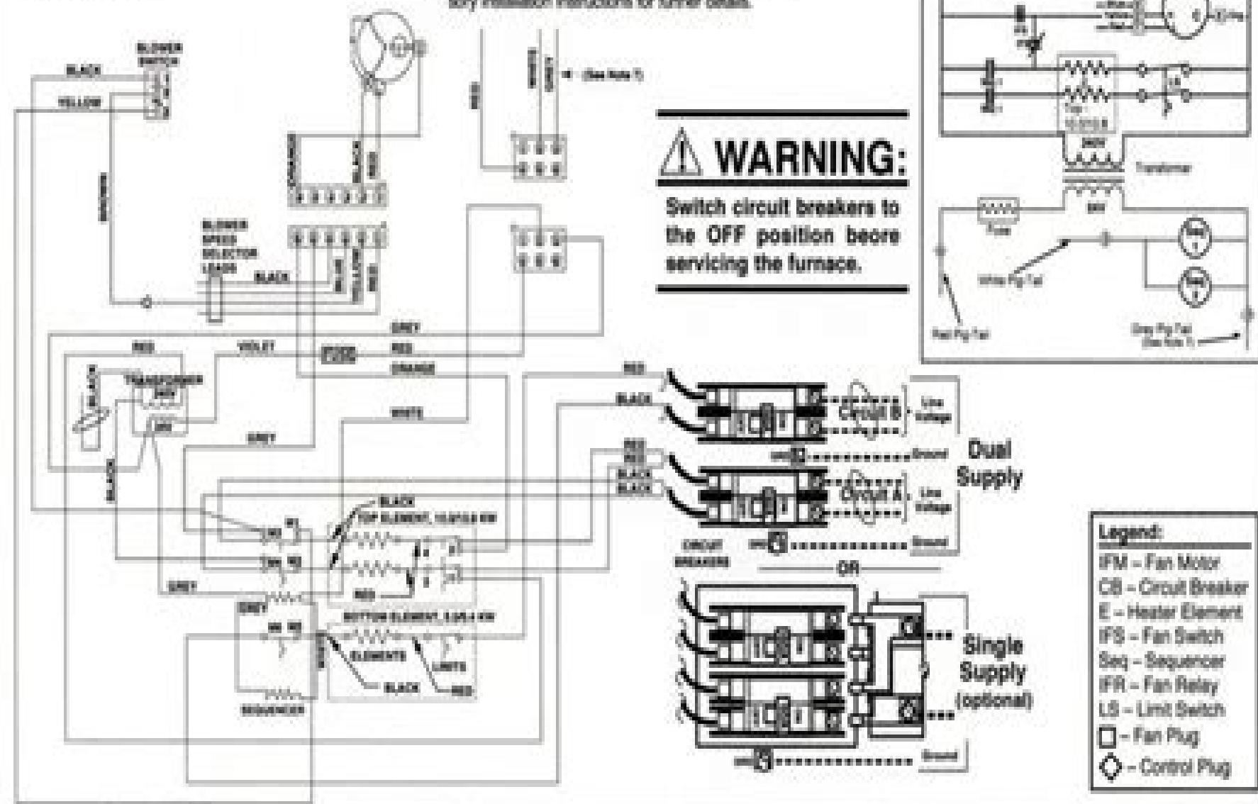
Figure 22. E22EH 015, 017 Wiring Diagrams
