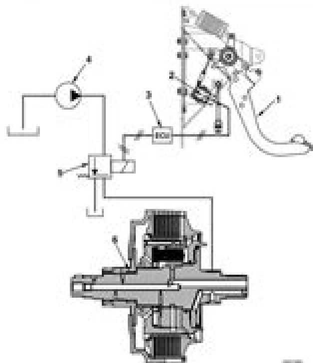
Fig. 11 - Main clutch actuation
