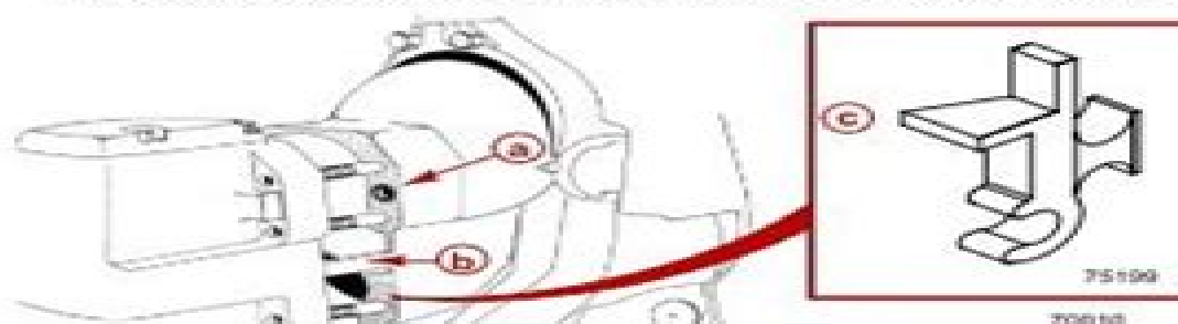
a - Gasket b - Shift Slide c - Shift Slide Stabilizer Tool
