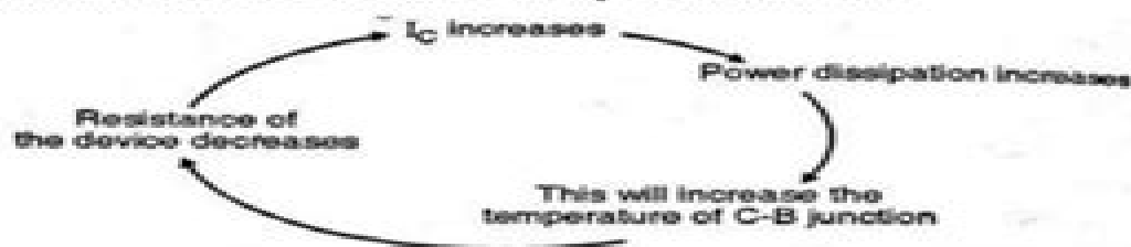
Fig. Thermal Runway
