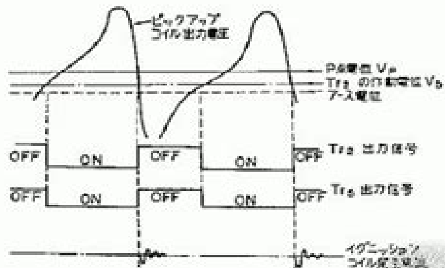
エンジン回転時の各トランジスタの作動
