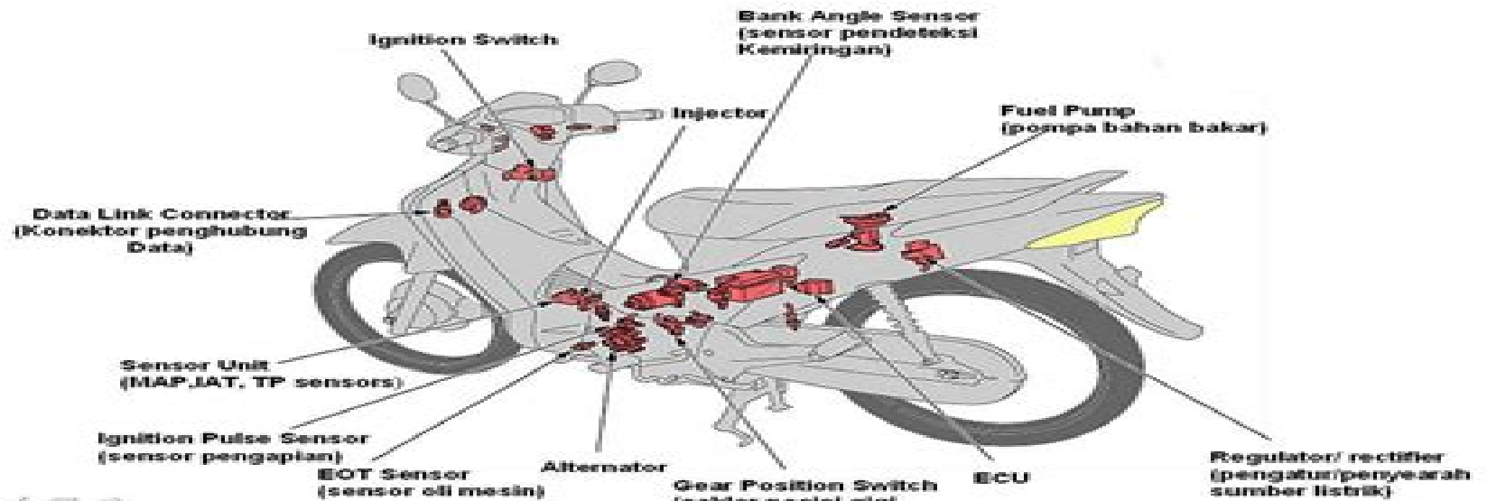
Gambar Komponen sistem EFI pada sepeda mesin Honda Supra X 125
