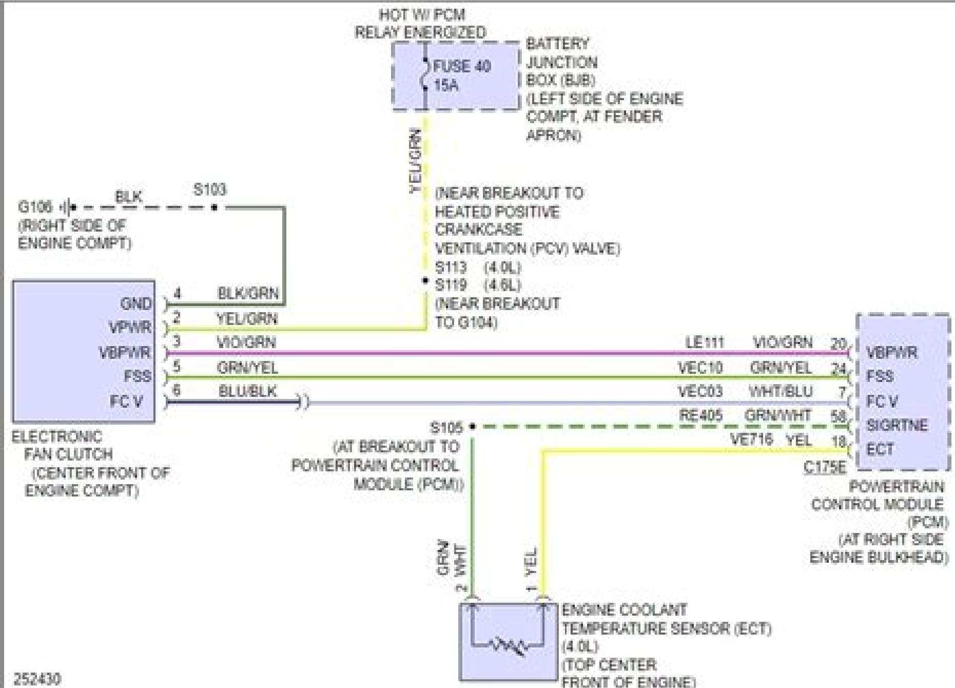
Fig 1: Cooling Fan Circuit
