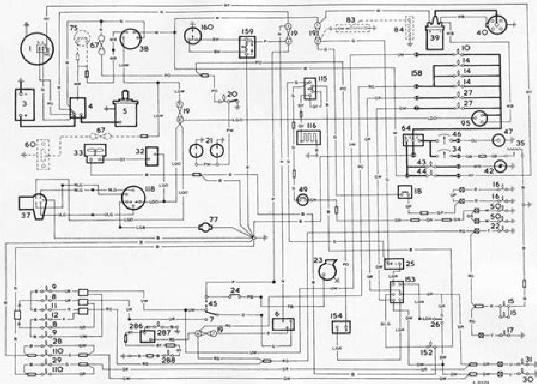
Wiring diagrams: 131 - Mini Special - 1977 to 78
