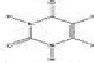
Uracil
