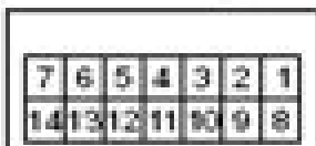
14P CONNECTOR (J802)
