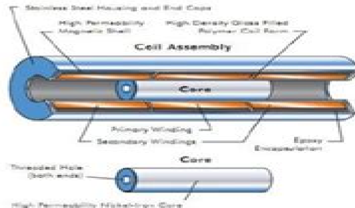
Fig: LVDT
