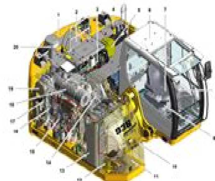
Fig. 3 Uppercarriage
