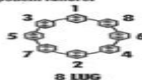
8 LUG
