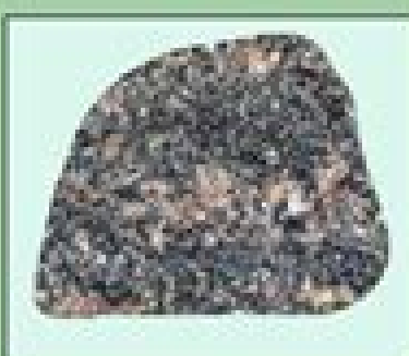
Migmatite
