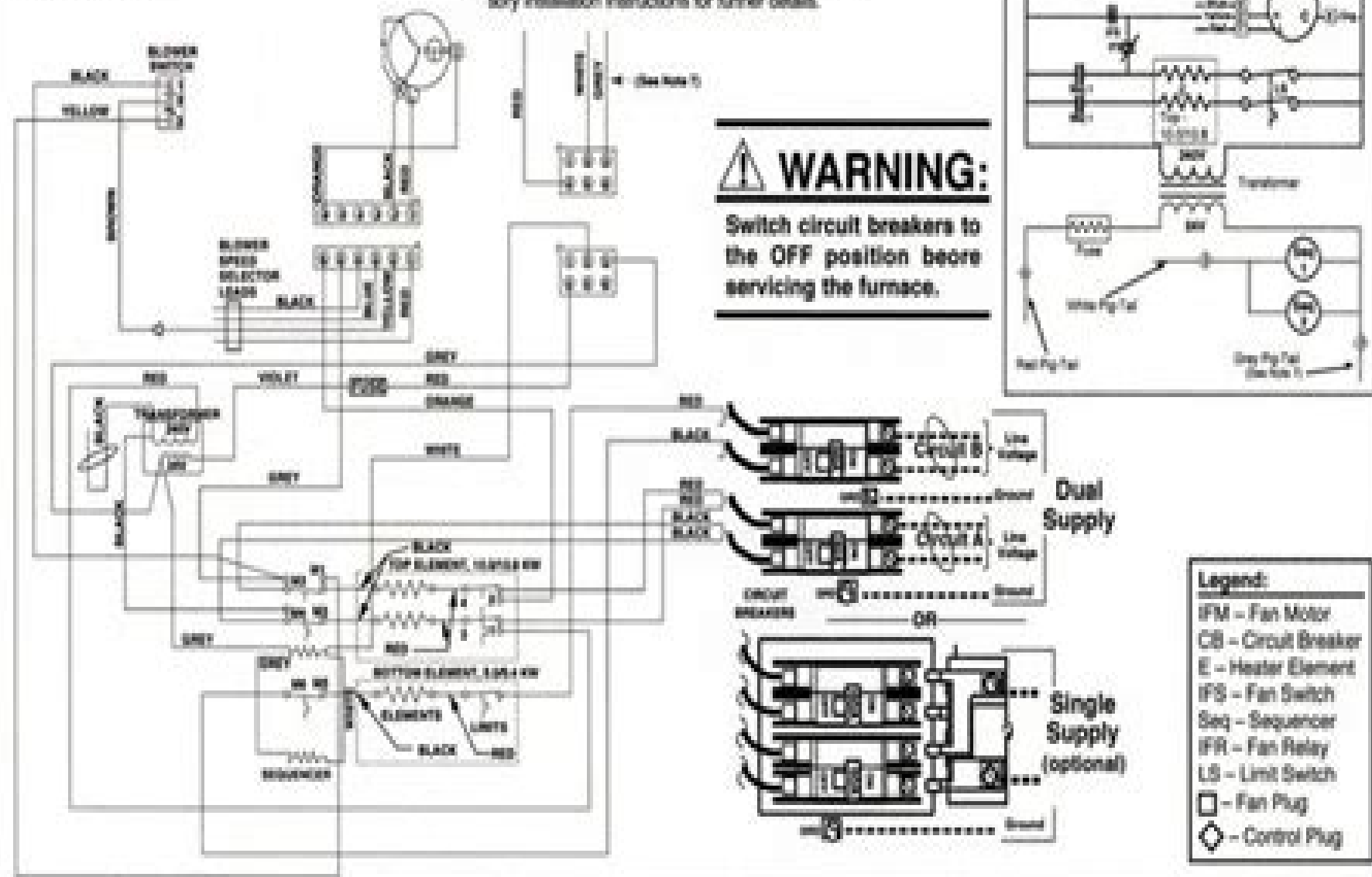
Figure 22. E22EH 015, 017 Wiring Diagrams
