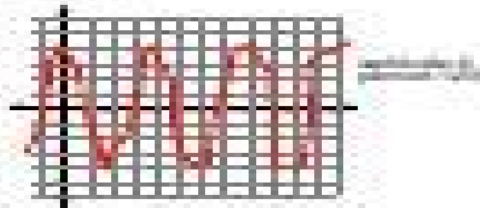
5) y = \sin(3x)
