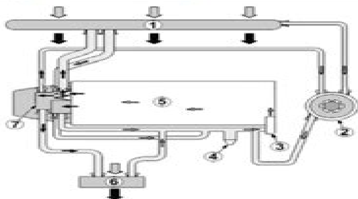
Complessivo sistema raffreddamento
