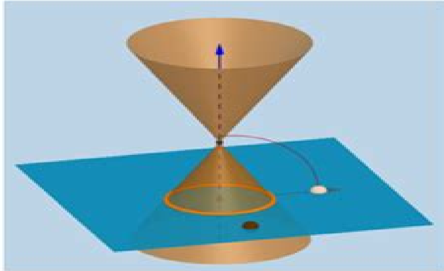
Circle
