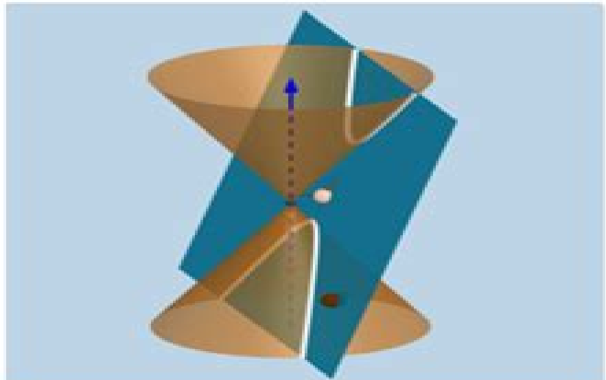
Hyperbola
