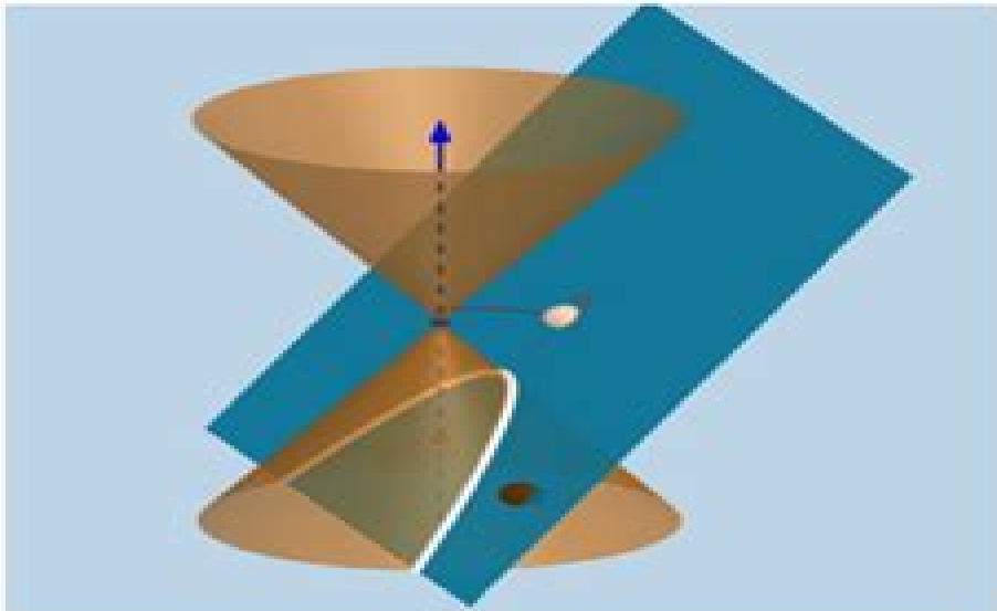
Parabola
