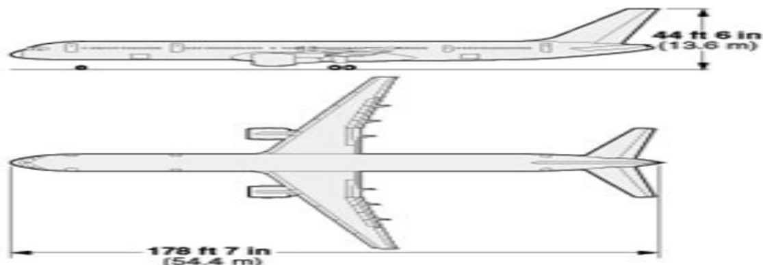
Boeing 757-300
