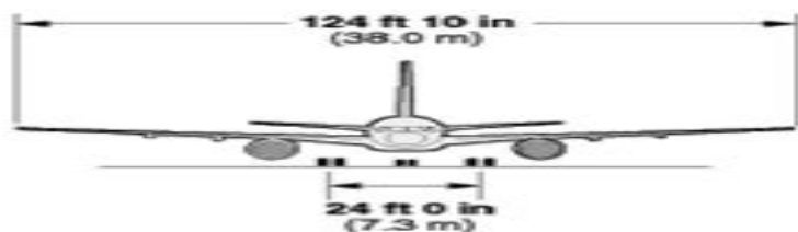
Boeing 757-200
