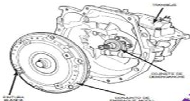
Fig. 13 Conjunto de embrague modular
