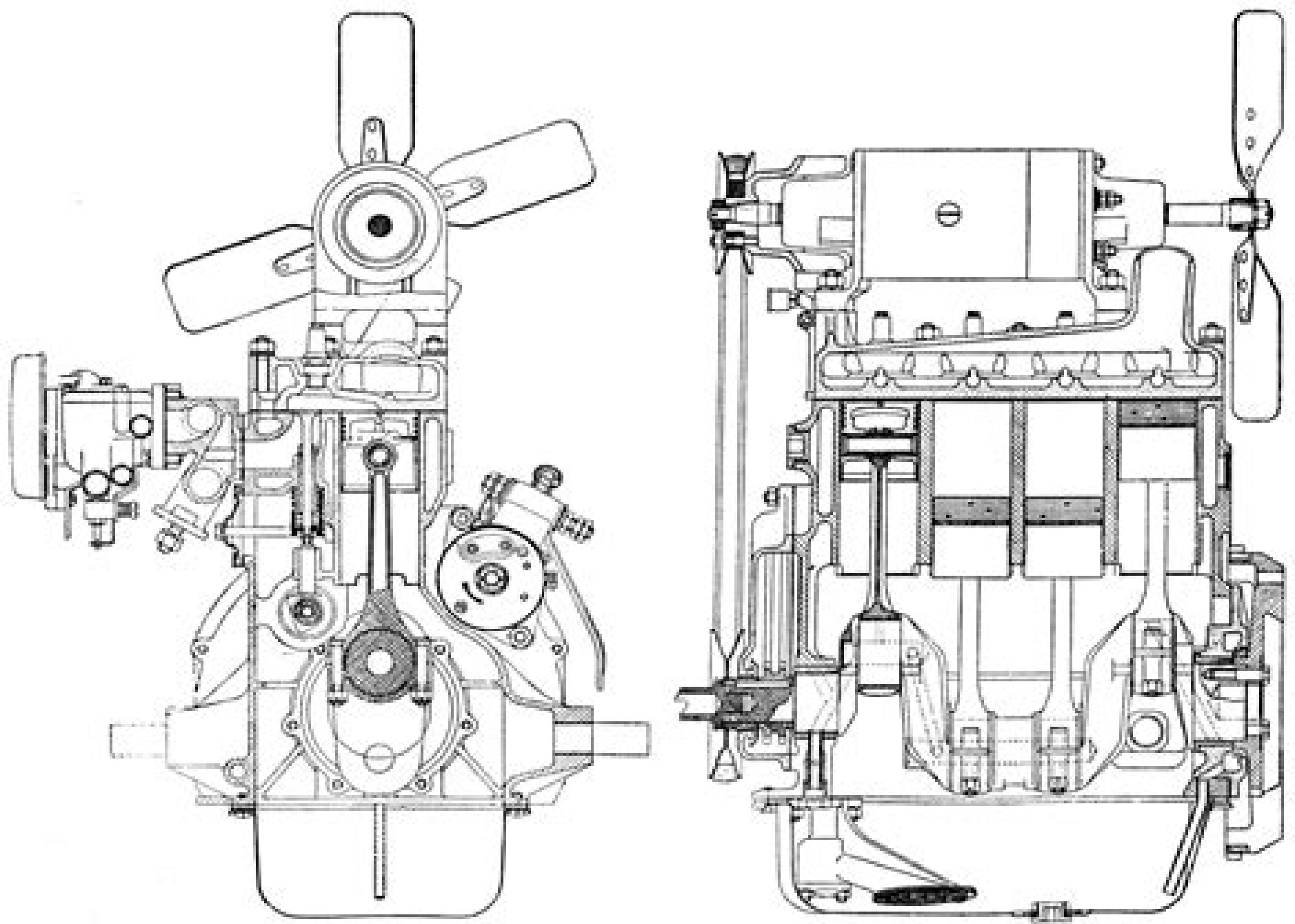
Fig. 75a—b. Langs- en dwarsdoorsnede van een Fiat 500.
