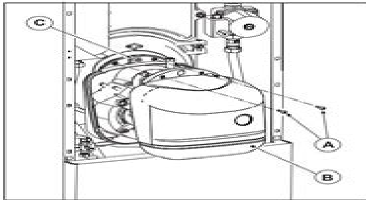
Fig. 35 - Desmontaje del quemador
