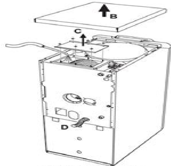
Fig. 37 - Limpieza del recuperador
