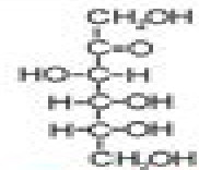
Fructose
