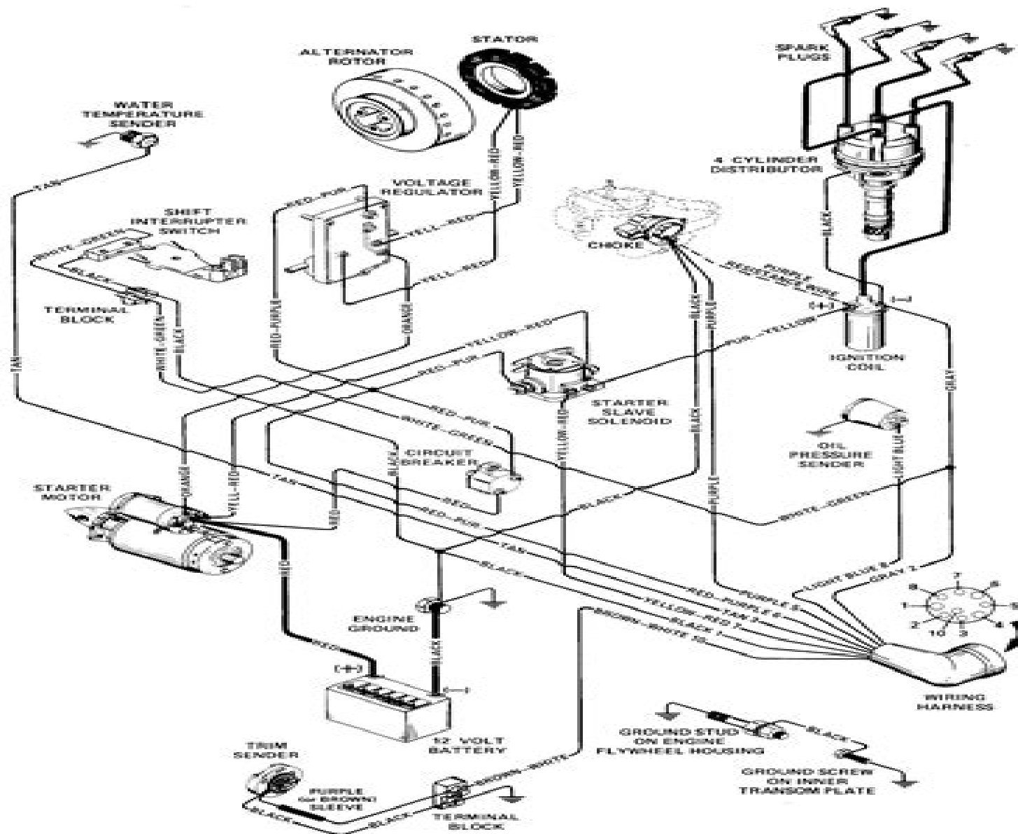
WIRING DIAGRAM 170/190
